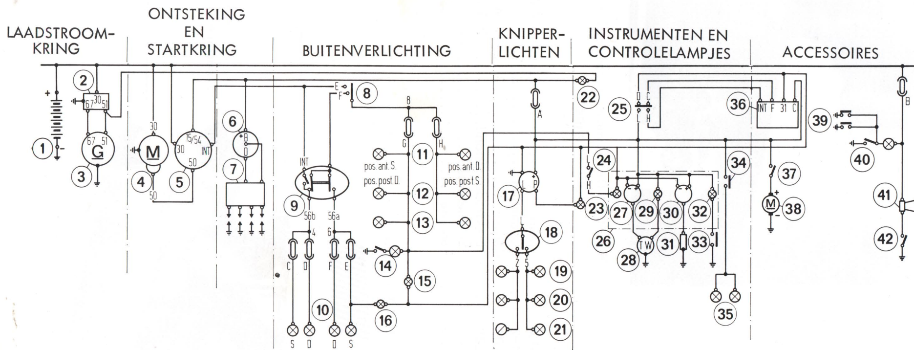
Fig.604 - Schema van elektrische installatie
